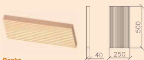
Doska 250x500x40
