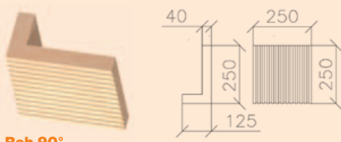
Roh 90° 125x250x250x40
