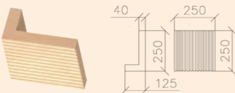
Roh 90° 125x250x250x40
