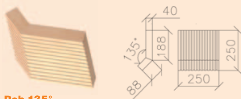
Roh 135° 125x250x250x40
