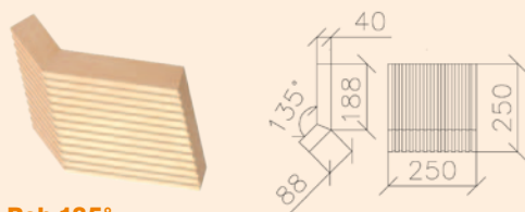
Roh 135° 125x250x250x40
