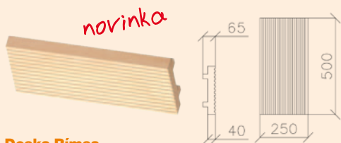
Doska Rímsa 250x500x40
