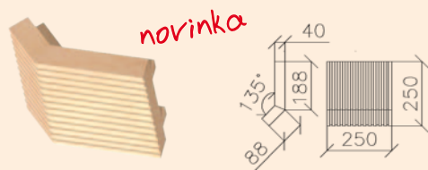
Roh 135° Rímsa 125x250x250x40
