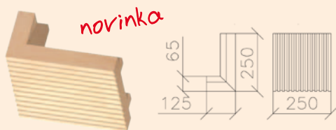
Roh 90° Rímsa 125x250x250x40
